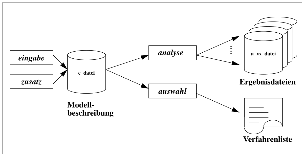
Abbildung 1: Programmaufbau des PEPSY-QNS
