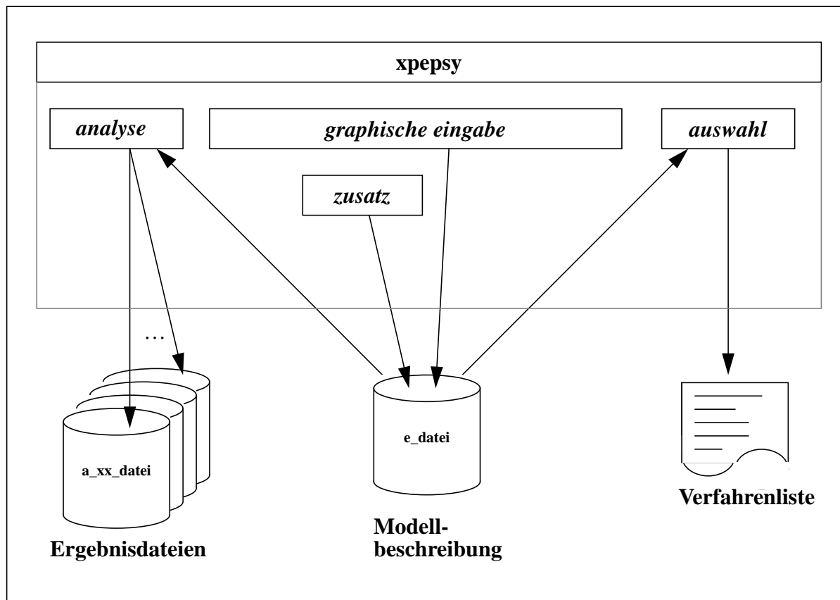
Abbildung 2: Die graphische Benutzungsschnittstelle XPEPSY
